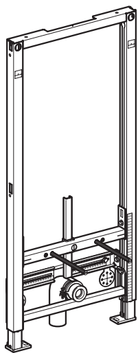
Монтажный элемент Geberit Duofix для подвесного биде
