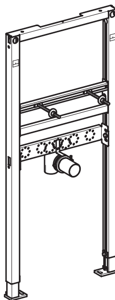
Монтажный элемент Geberit Duofix для умывальника
